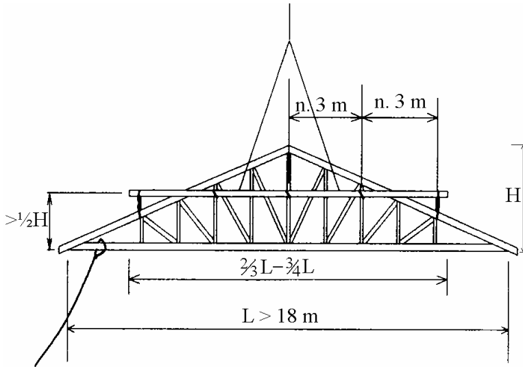
Kuva 5. Nosto palkin kanssa viidestä pisteestä tuetuna, kun L > 18\text{ m} .
