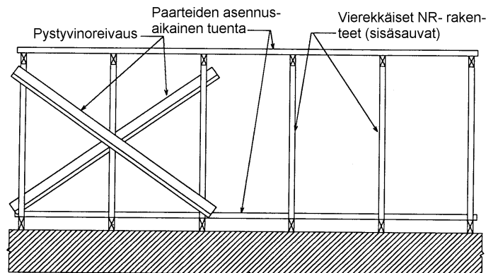
Kuva 8. Asennusaikainen pystyvinoreivaus. X-tukien välinen etäisyys on kannattimien suunnassa enintään 2,5 m.
